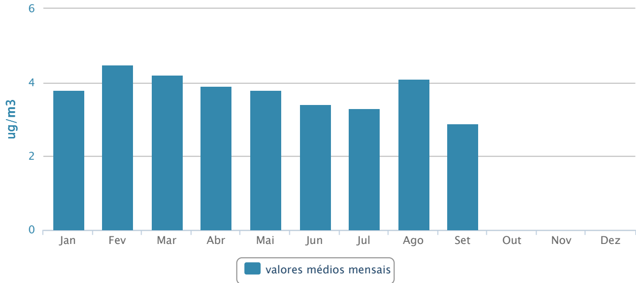
Registos de monitorização de qualidade do ar da Ribeira Grande para o poluente NOx em 2022
