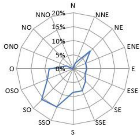
Direção do Vento - Angra do Heroísmo
