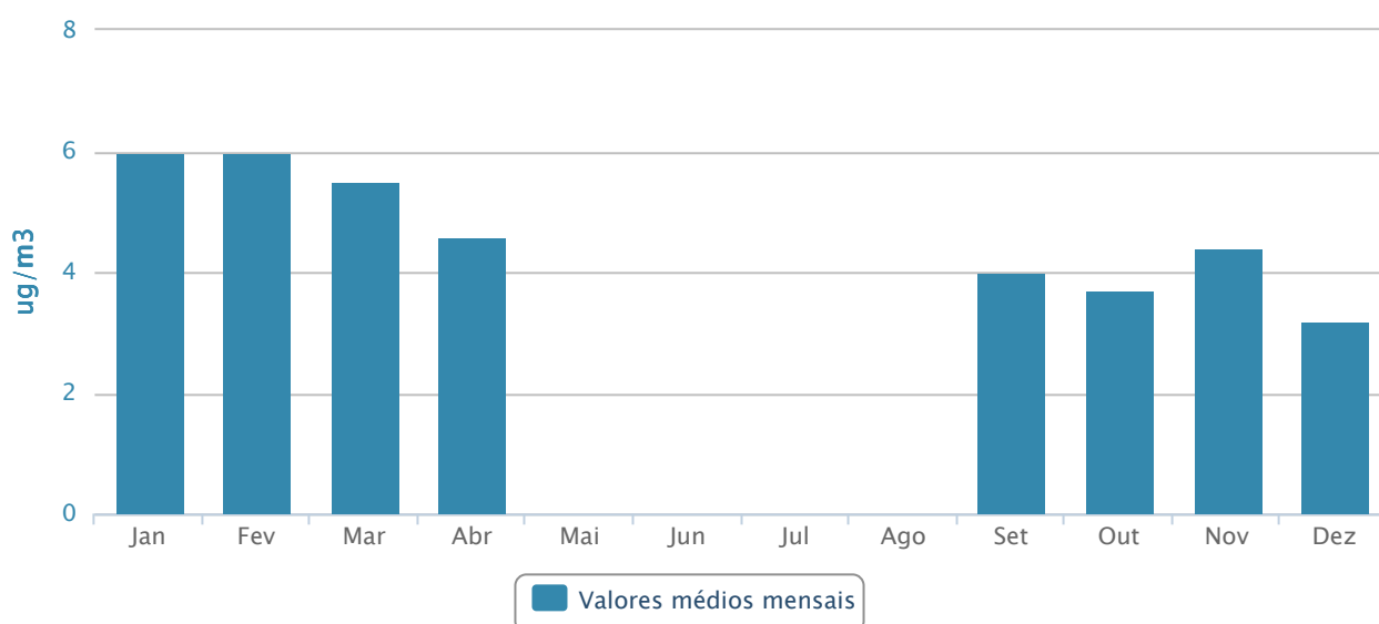
Registos de monitorização de qualidade do ar de Angra do Heroísmo para o poluente NO 2 em 2022
