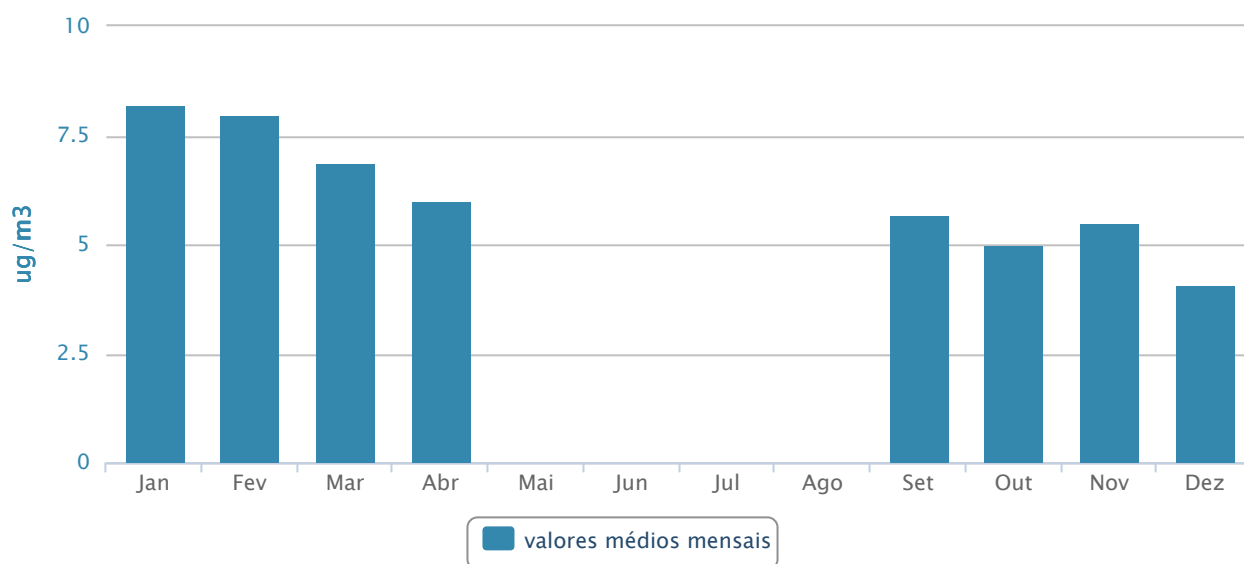
Registos de monitorização de qualidade do ar de Angra do Heroísmo para o poluente NOx em 2022
