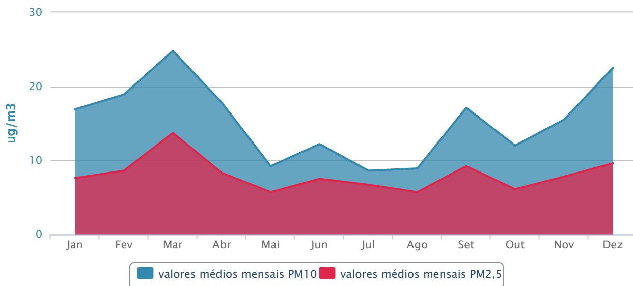
Registos de monitorização de qualidade do ar de Ponta Delgada para o poluente partículas em suspensão em 2022
