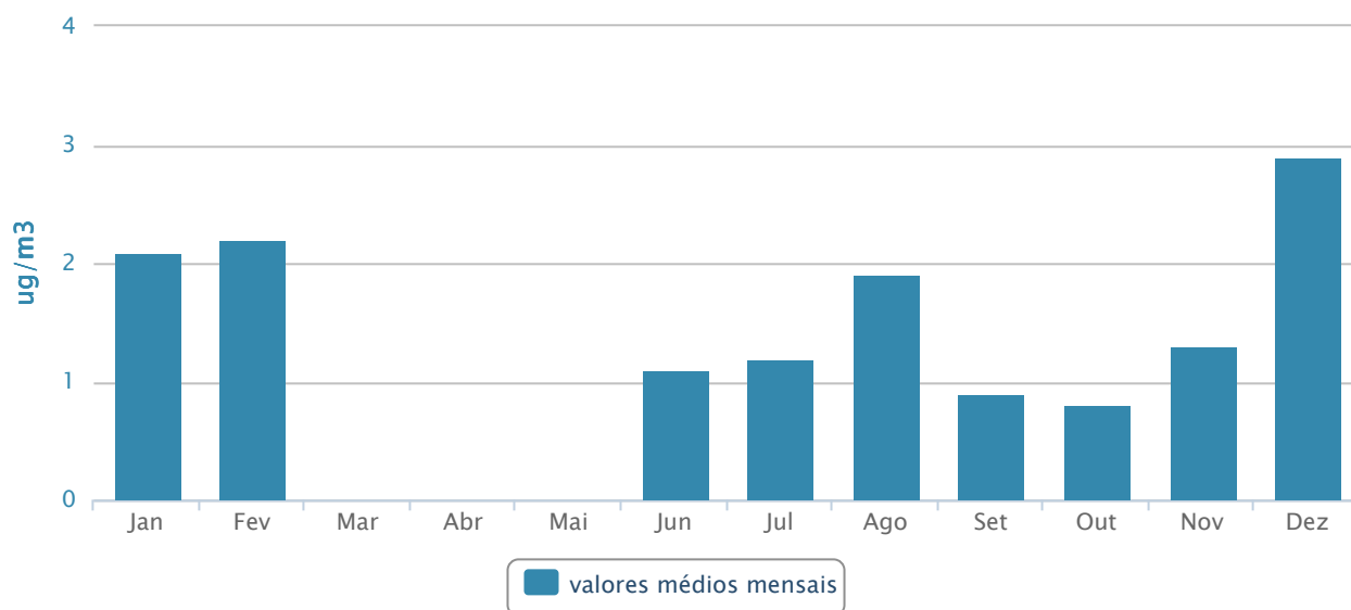
Registos de monitorização de qualidade do ar do Faial para o poluente NOx em 2022
