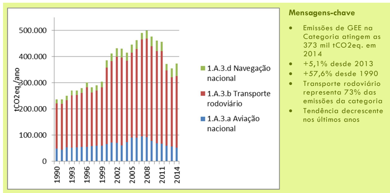
Figura 16: Emissões da Queima de Combustíveis nos Transportes
