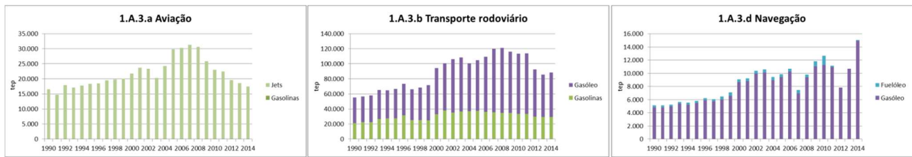
Figura 11: Consumos de Combustíveis Usados – 1.A.3 Transportes
