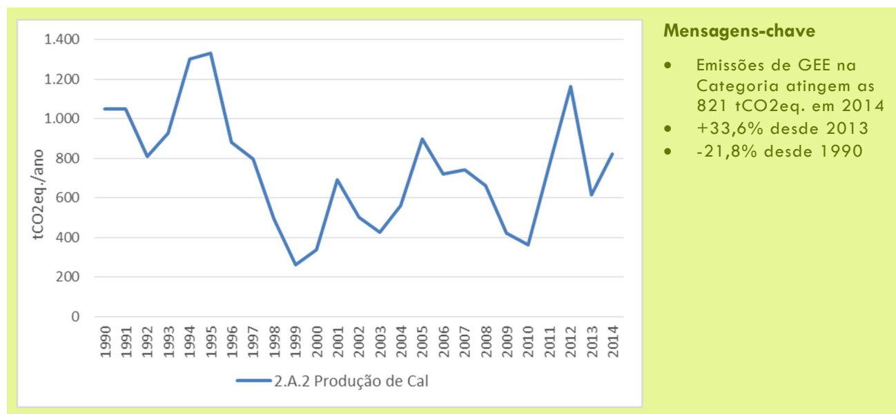
Figura 21: Emissões da Utilização de Carbonatos na Produção de Cal
