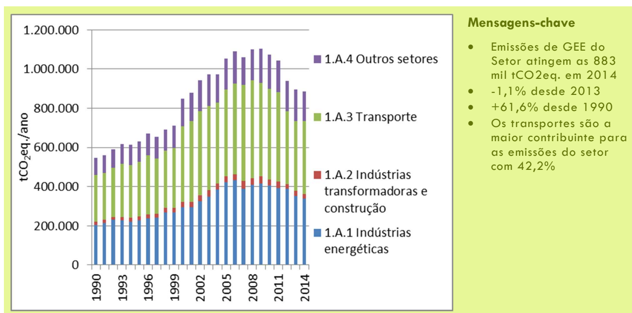
Figura 7: Evolução das Emissões do Setor Energia
