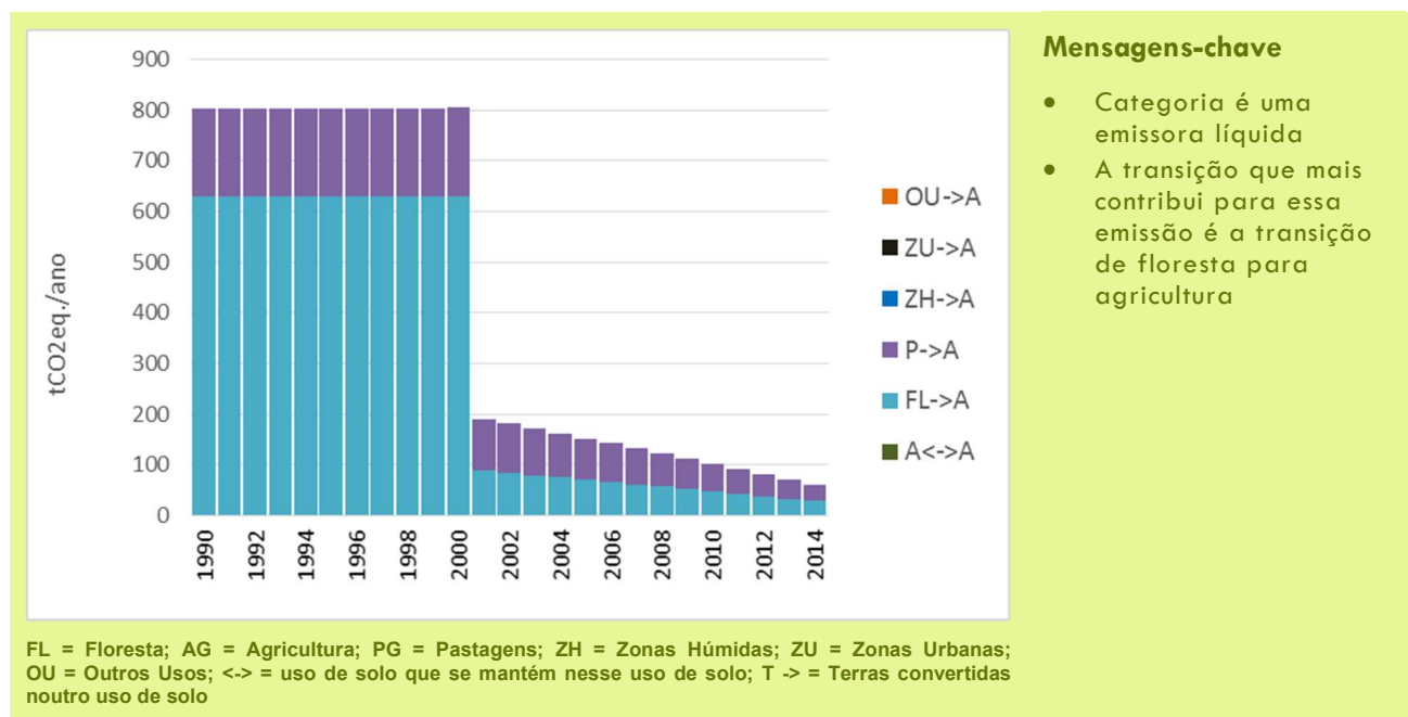
Figura 43: Emissões / Sequestro da Categoria 4B Agricultura: por subcategoria
