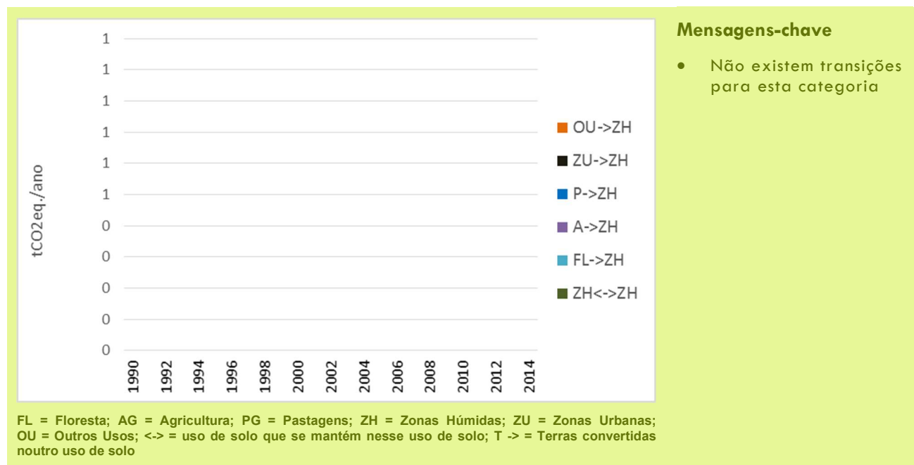
Figura 47: Emissões / Sequestro da Categoria 4D Zonas Húmidas: por subcategoria
