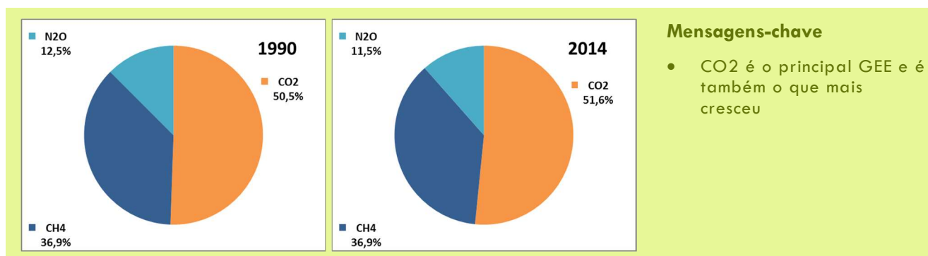
Figura 3: Perfil de Emissões por Gás de Efeito de Estufa na RAA em 1990 e 2014
