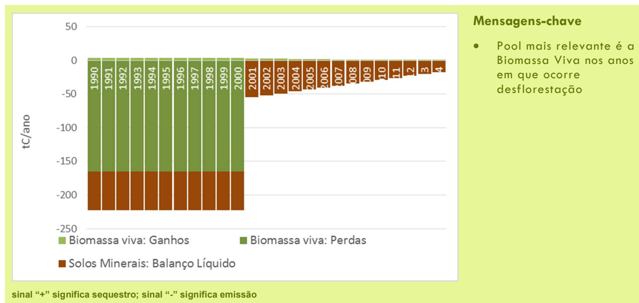
Figura 44: Emissões / Sequestro da Categoria 4B Agricultura: por pool
