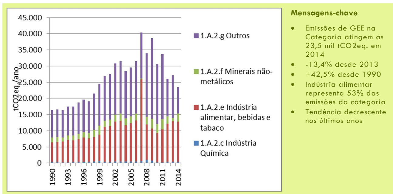
Figura 15: Emissões da Queima de Combustíveis na Indústria Transformadora e Construção
