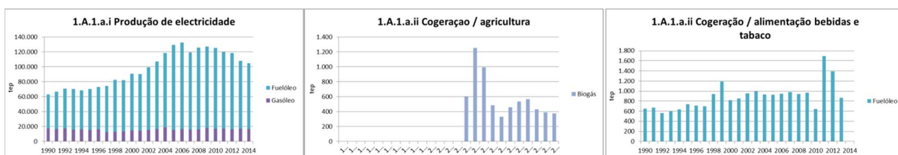
Figura 9: Consumos de Combustíveis Usados – Setor 1.A.1 Indústrias da Energia
