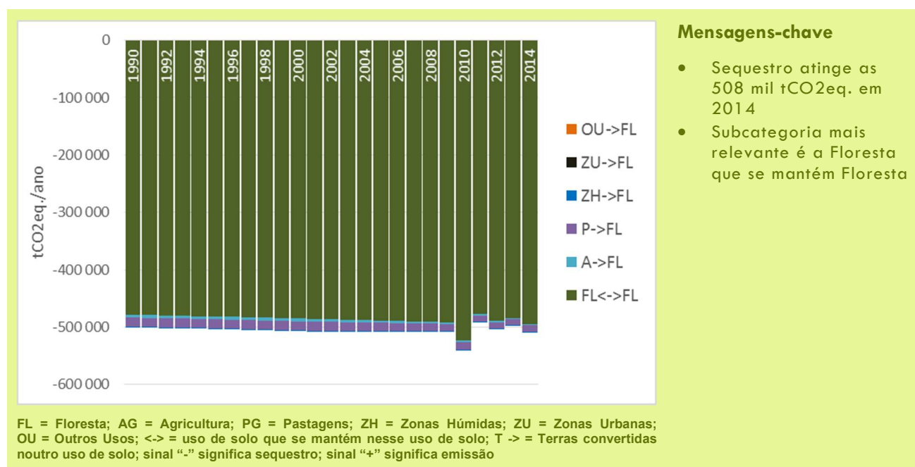
Figura 41: Emissões / Sequestro da Categoria 4A Floresta: por subcategoria
