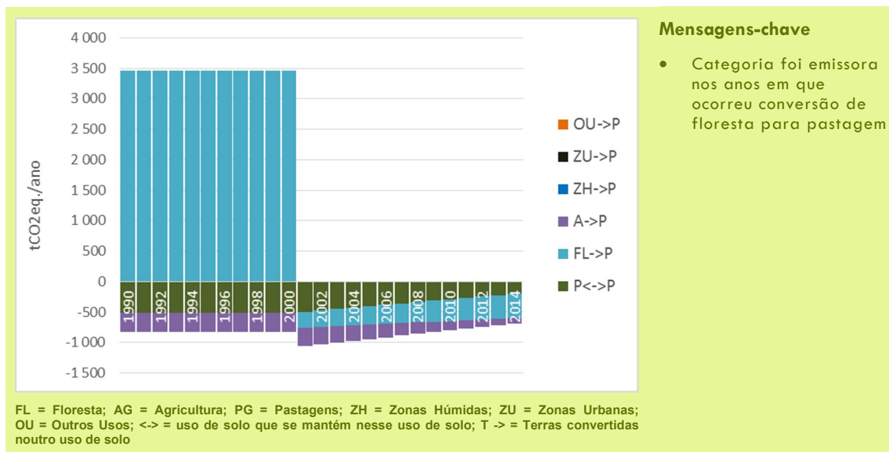
Figura 45: Emissões / Sequestro da Categoria 4C Pastagens: por subcategoria
