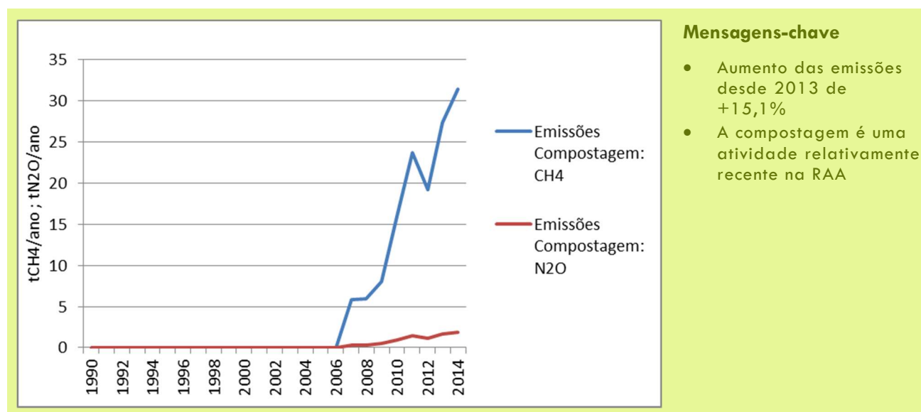
Figura 62: Emissões de Metano e Óxido Nitroso de Compostagem
