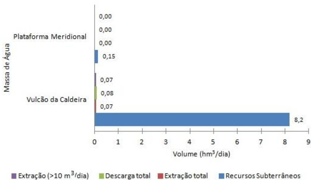
Figura 3.4.23 | Gráfico comparativo do volume médio extraído nos pontos de água com caudal superior a 10 m³/dia, face à descarga natural total, às extrações totais efetuadas e aos recursos hídricos subterrâneos globais.
