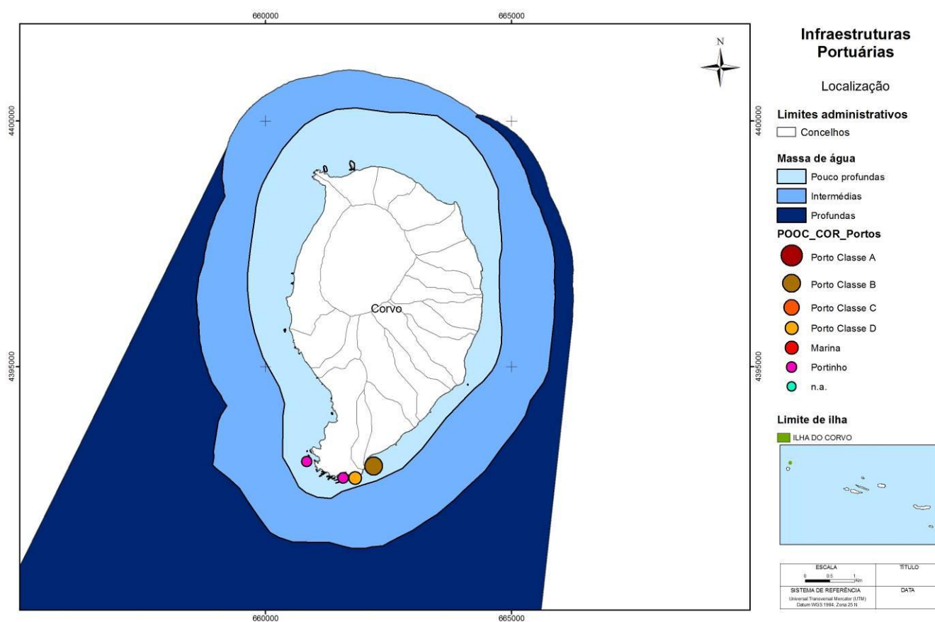
Figura 3.4.12 | Localização das infraestruturas portuárias.
