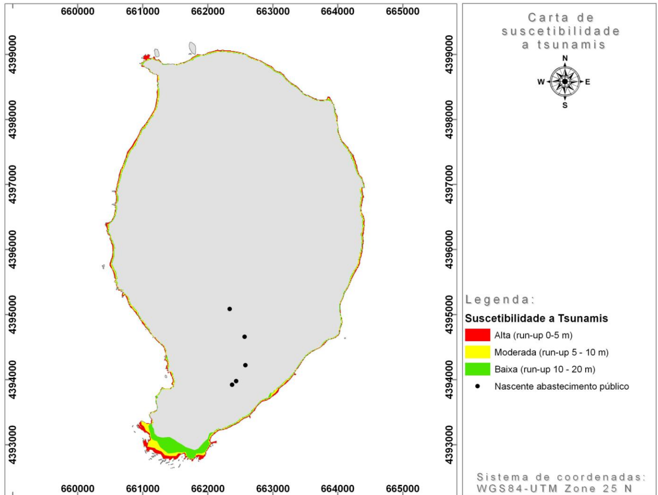
Figura 2.9.16 | Carta de suscetibilidade a tsunamis . O run-up máximo de cada classe considerada corresponde à cota máxima da área inundada.
