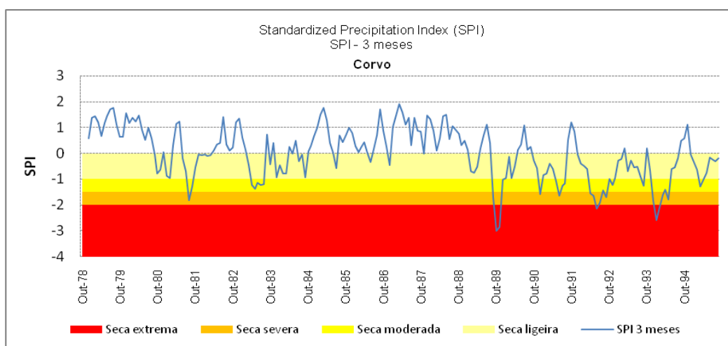
Figura 2.9.8 | Resultados do índice SPI para a escala temporal a 3 meses para a ilha do Corvo (período de outubro de 1978 a setembro de 1995).
