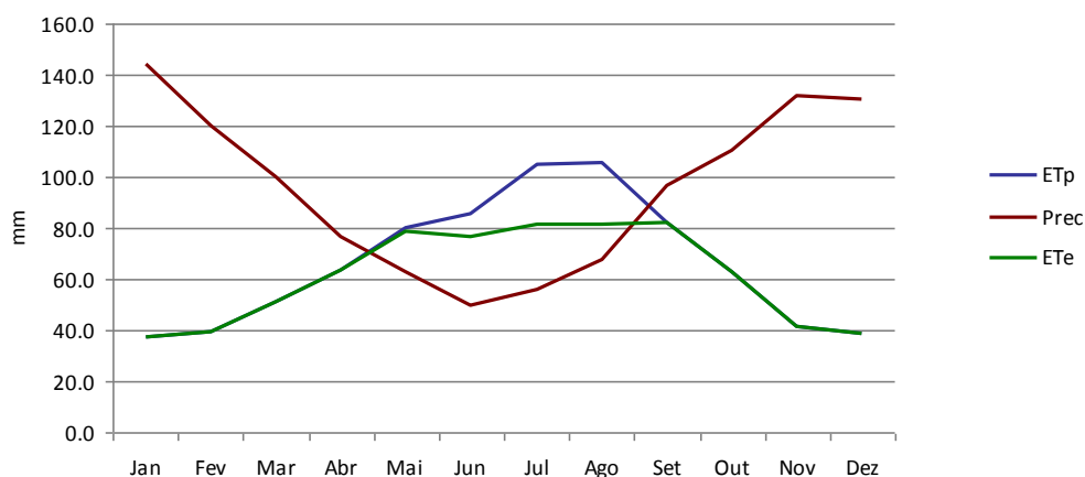
Figura 2.2.2 | Balanço Hídrico Sequencial para a ilha do Corvo.
