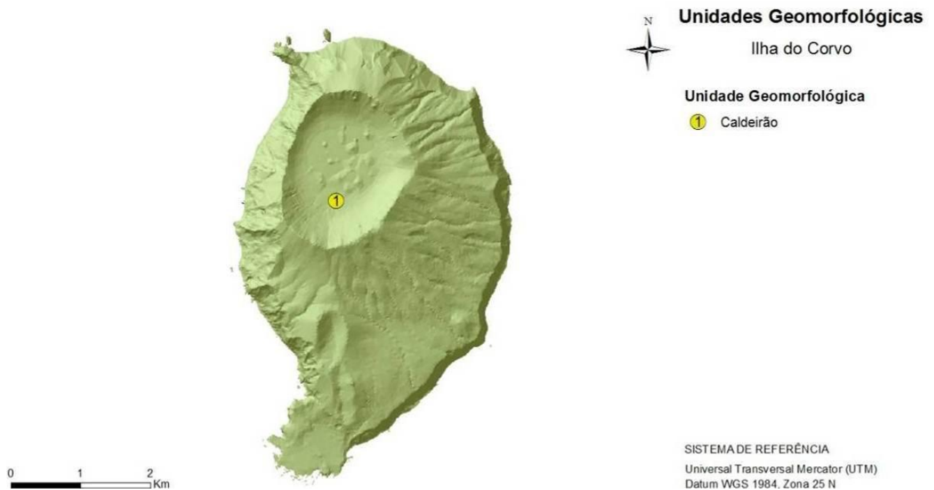
Figura 2.3.13 | Carta das unidades geomorfológicas da ilha do Corvo.
