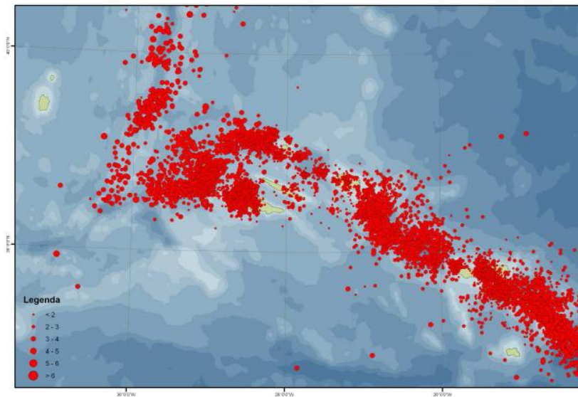
Figura 2.9.15 | Carta epicentral dos eventos registados entre 1997 e 2009.
