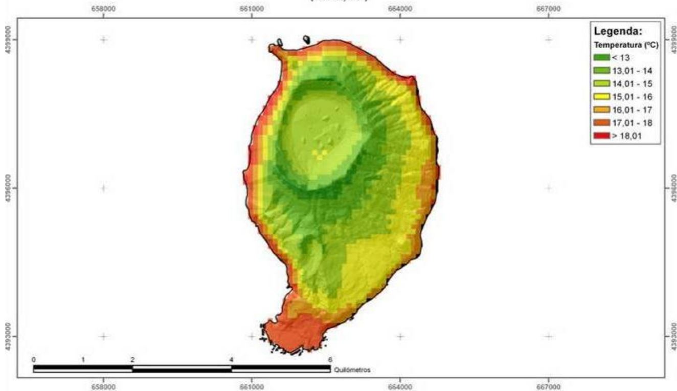
Figura 2.2.12 | Modelo CIELO – expressão espacial da temperatura na ilha do Corvo.
