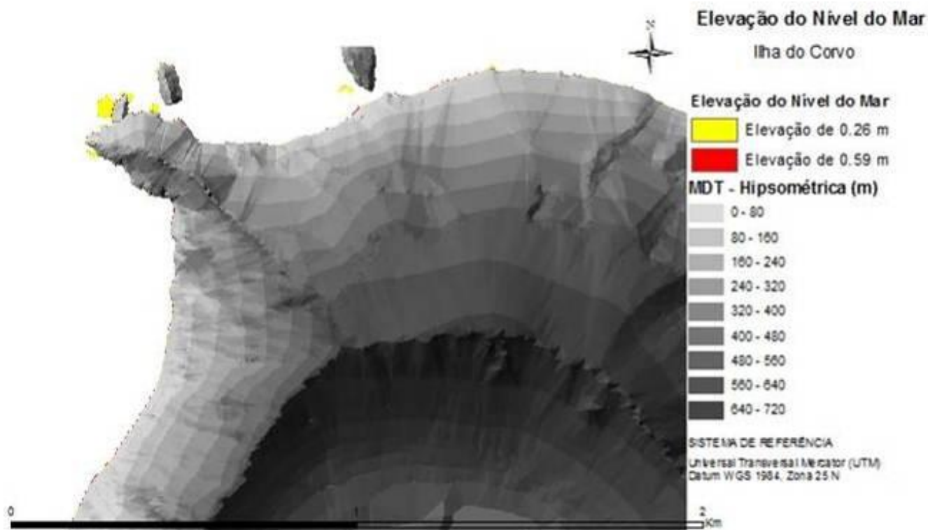
Figura 2.9.4 | Elevação do nível do mar na Ponta do Marco da ilha do Corvo.
