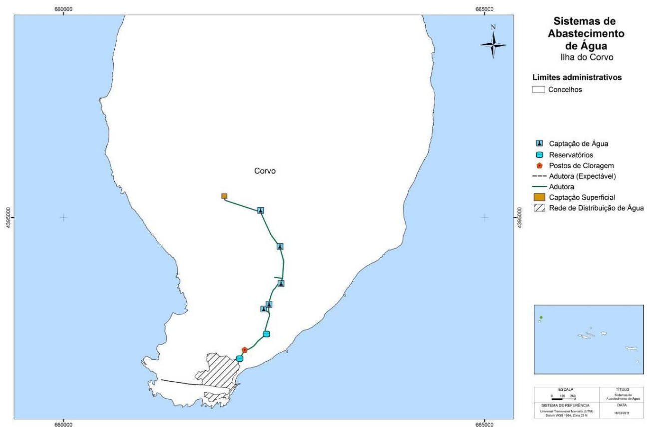
Figura 2.8.1 | Representação gráfica do sistema de abastecimento de água da ilha do Corvo.
