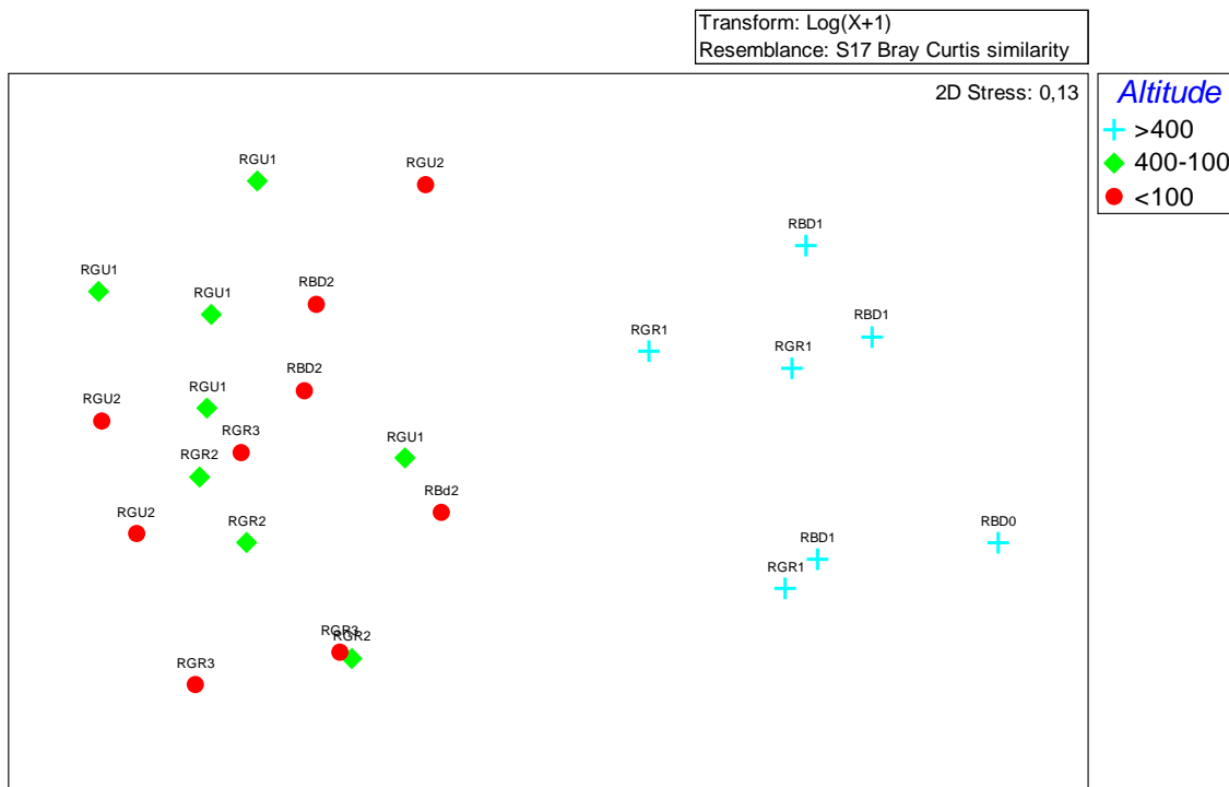
Figura 3.1.2 | Análise de ordenação por nMDS das comunidades de diatómeas bentónicas das ribeiras consideradas de referência na Região Hidrográfica Açores, com sobreposição do fator altitude (ver códigos do locais de amostragem no Quadro 4.1.1).
