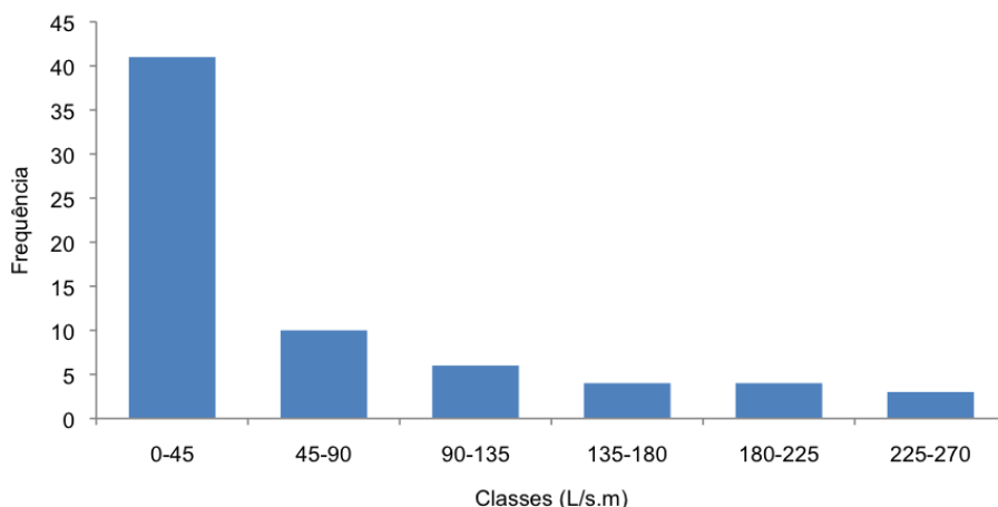
Figura 2.3.16 | Histograma relativo à distribuição de valores de caudal específico na RH9.
