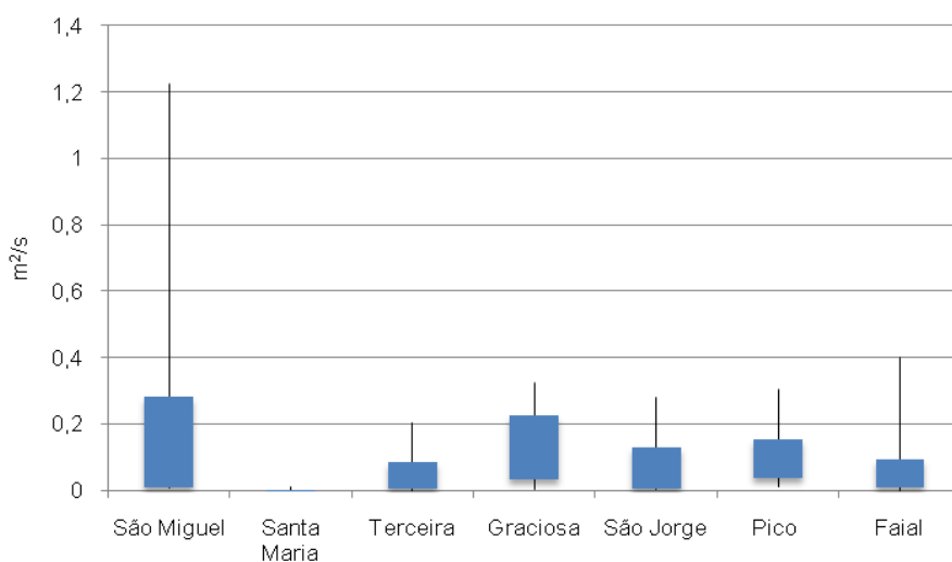
Figura 2.3.17 | Diagrama de caixas (box plot) relativo aos valores de transmissividade na RH9.
