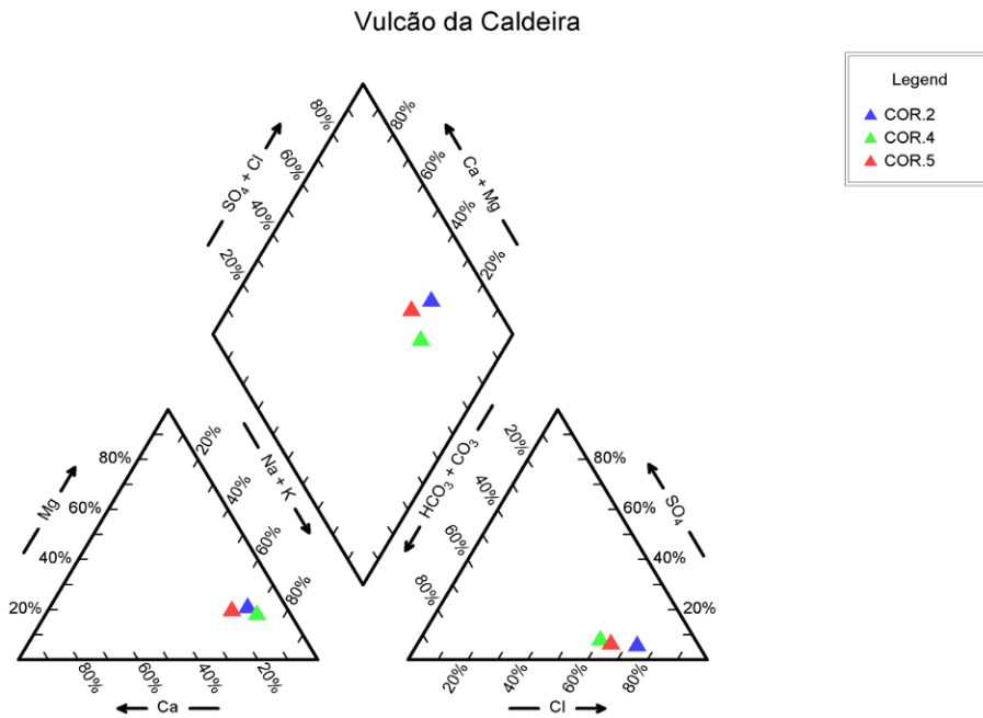
Figura 5.1.18 | Diagrama de Piper relativo à mediana da composição química da água monitorizada na massa de água Vulcão da Caldeira. (Triângulos – Nascentes).
