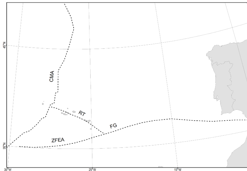
Figura 2.3.2 | Principais estruturas tectónicas da região dos Açores. Legenda: CMA - Crista Média Atlântica; ZFEA - Zona de Fratura Este dos Açores; FG - Falha Gloria; RT - Rift da Terceira, ZFOA - Zona de Fratura Oeste dos Açores.
