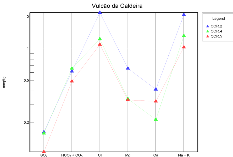
Figura 5.1.19 | Diagrama de Schoeller relativo à mediana da composição química da água monitorizada na massa de água Vulcão da Caldeira. (Triângulos – Nascentes).
