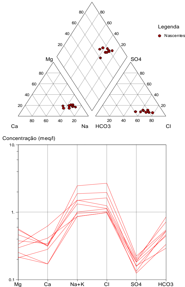
Figura 2.3.23 | Diagramas de Piper e de Schoeller relativos à composição química da água captada nas nascentes na ilha do Corvo.
