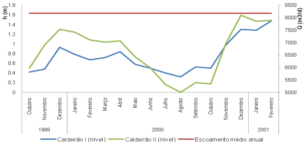
Figura 3.4.2 | Variação de nível na lagoa do Caldeirão.
