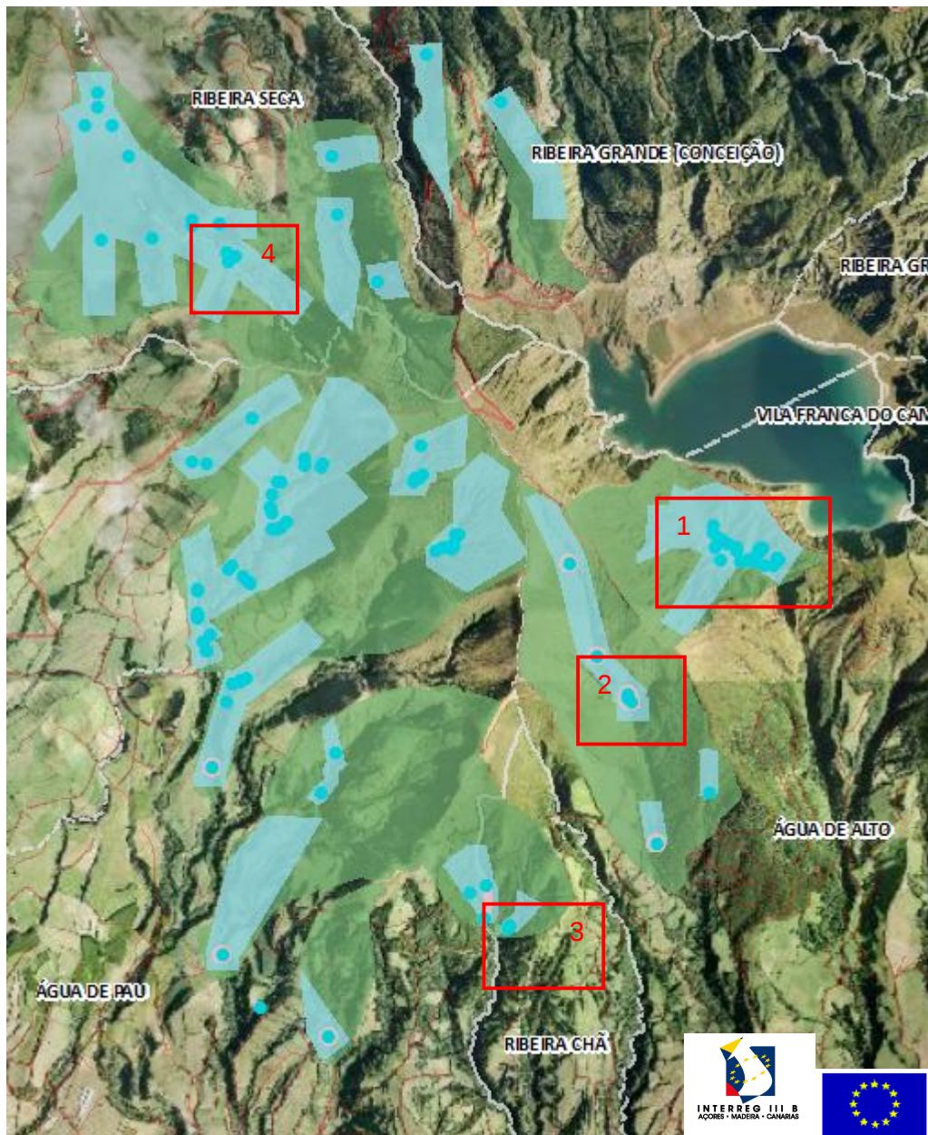
Ilustração 1 – Exemplos da forte sobreposição de elementos de alguns clusters de captações de água de abastecimento público.
