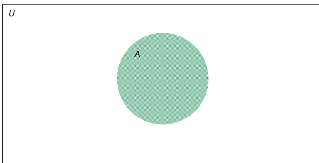
Ilustração 2 – Diagrama de Venn.
