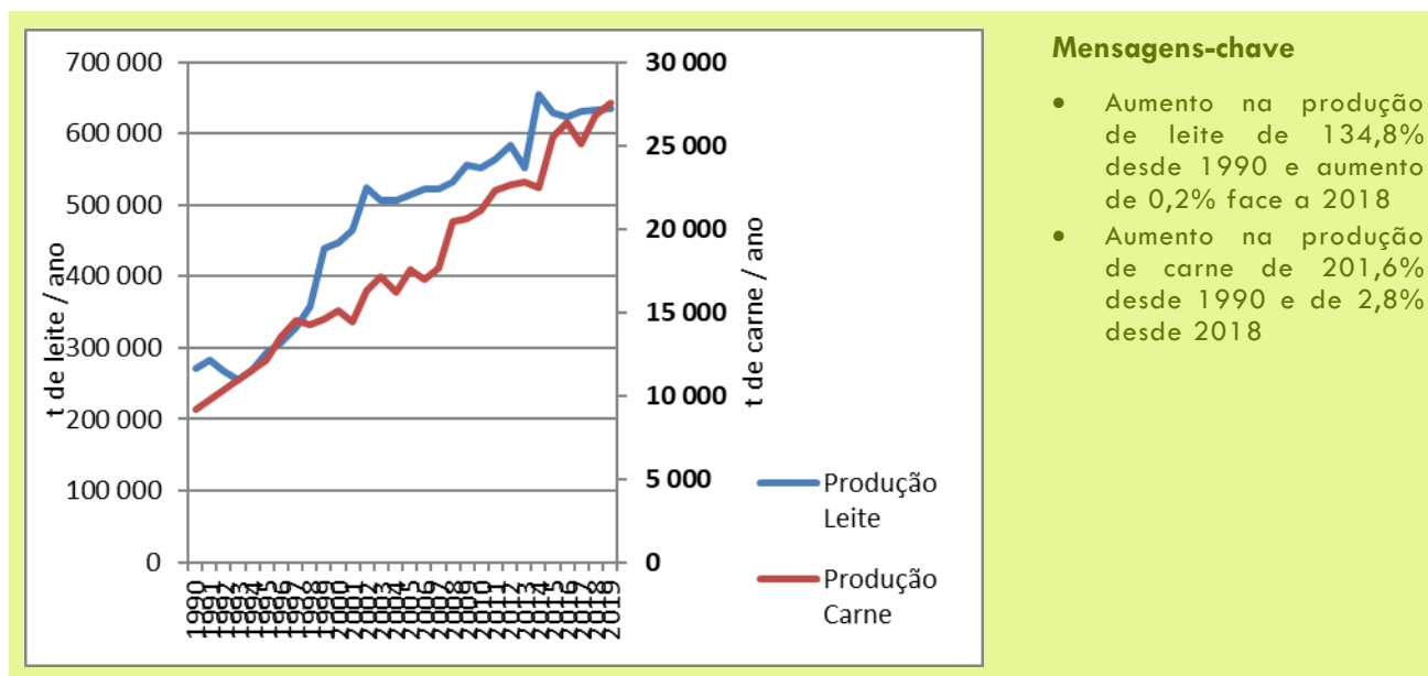
Figura 67: Produção de Carne e de Leite na RAA
