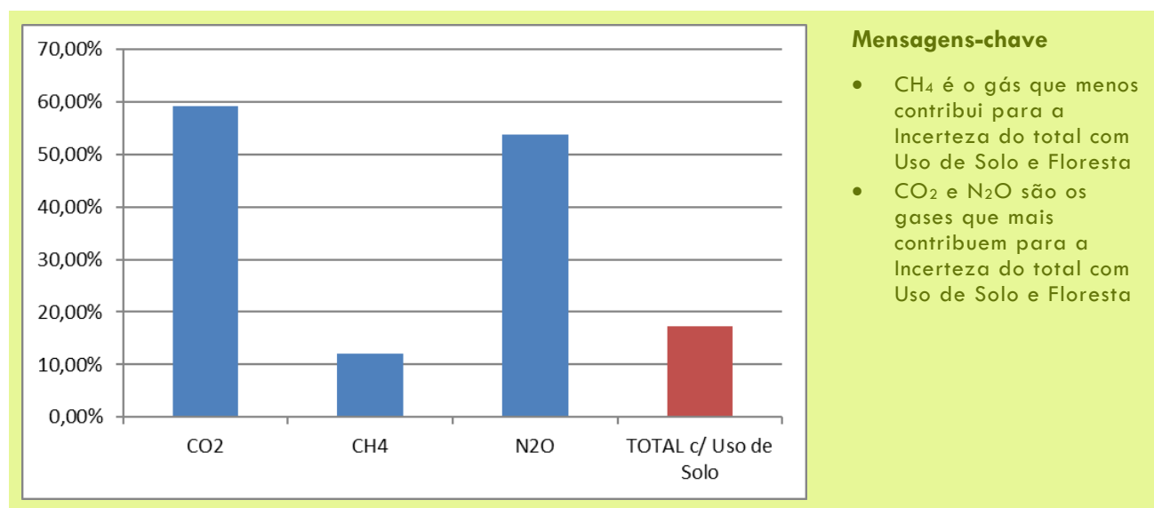
Figura 71: Distribuição da Incerteza Com Uso de Solo por Gás com efeito de Estufa em 2019
