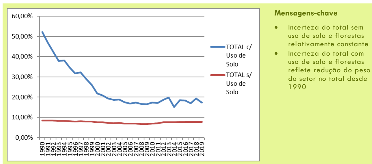
Figura 73: Evolução da Incerteza do IRERPA 1990-2019
