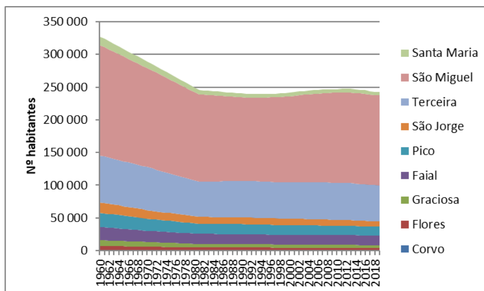
Figura 54: Evolução de População na RAA
