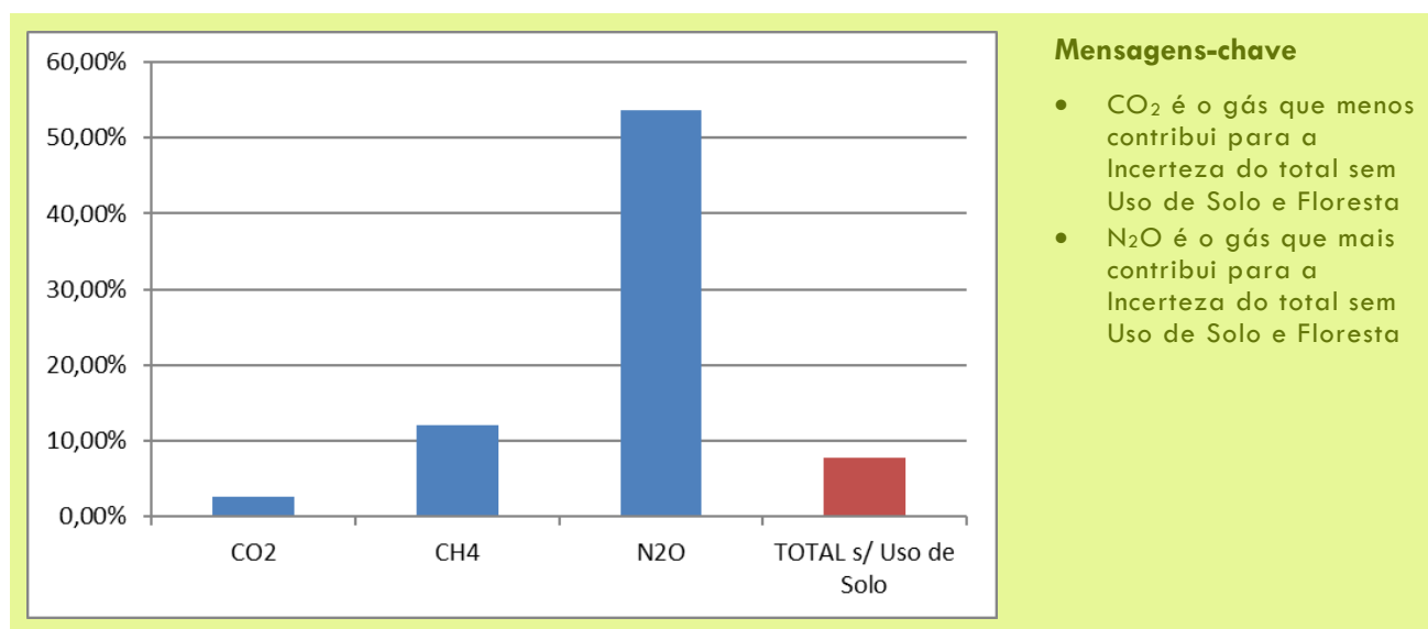
Figura 72: Distribuição da Incerteza Sem Uso de Solo por Gás com efeito de Estufa em 2019
