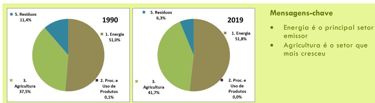
Figura 2: Perfil de Emissões por Setor na RAA em 1990 e 2019
