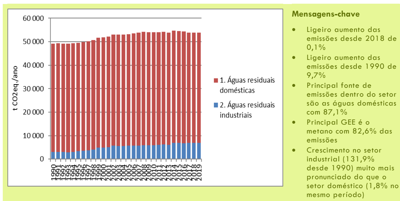
Figura 69: Emissões do Tratamento de Águas Residuais
