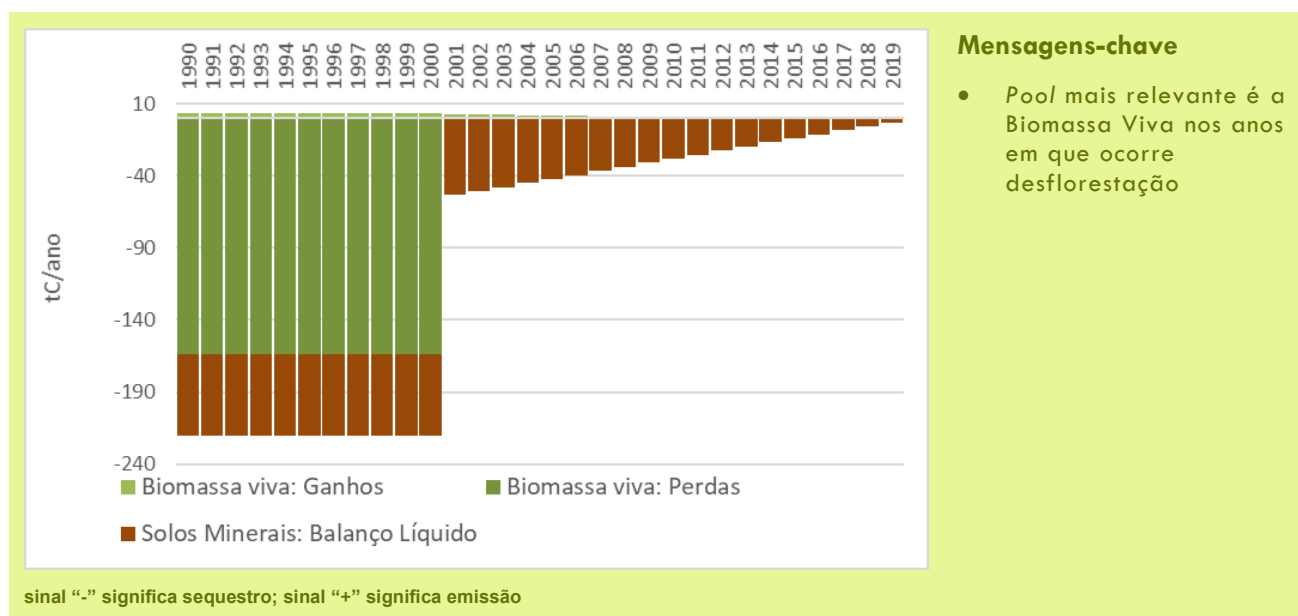
Figura 45: Emissões / Sequestro da Categoria 4B Agricultura: por pool
