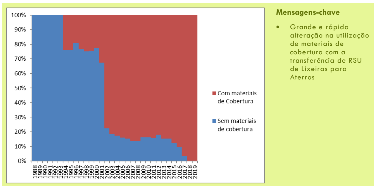
Figura 58: Distribuição Percentual dos Resíduos Depositados com e sem Utilização de Materiais de Cobertura
