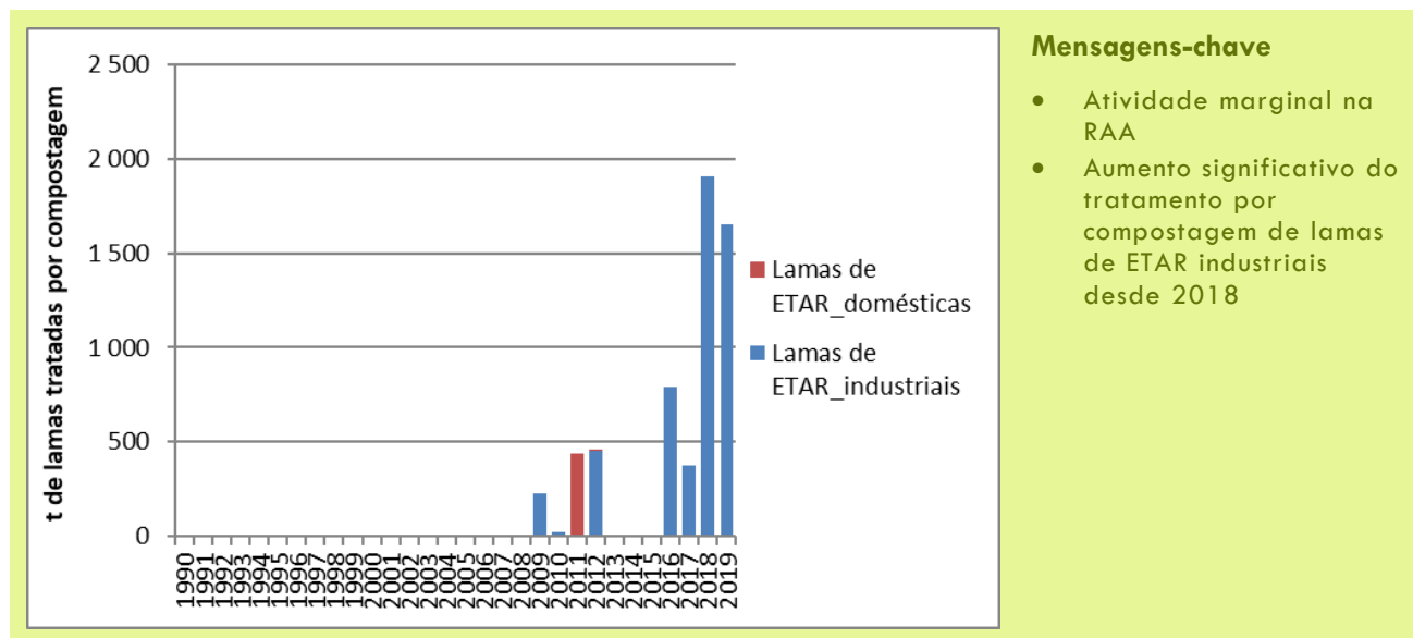
Figura 62: Evolução da Produção de Lamas do Tratamento de Águas Residuais Tratados por Compostagem
