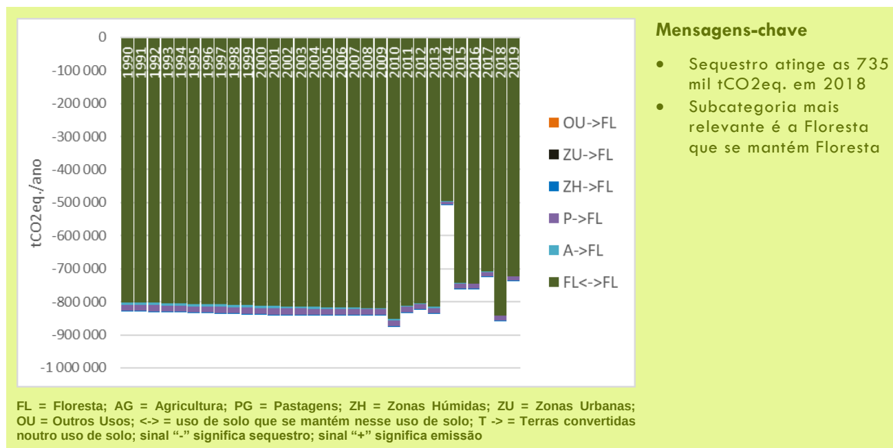
Figura 42: Emissões / Sequestro da Categoria 4A Floresta: por subcategoria
