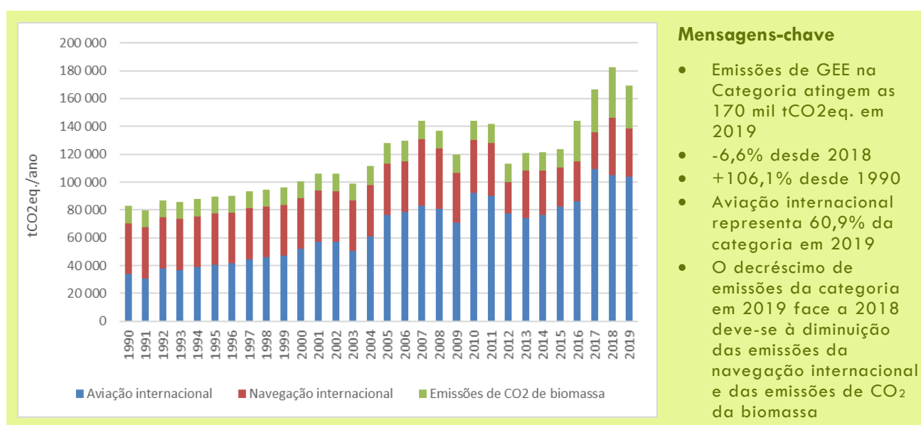
Figura 18: Emissões da Queima de Combustíveis na Categoria “Para Memória”
