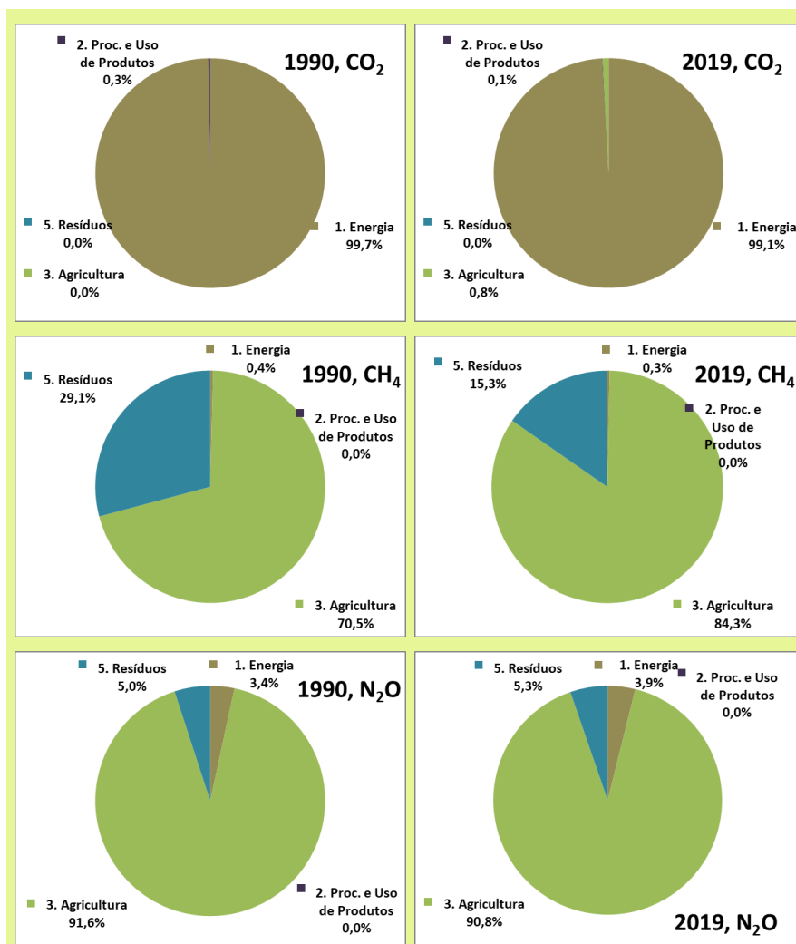
Figura 4: Perfil de Emissões por Gás com Efeito de Estufa e por Setor na RAA em 1990 e 2019
