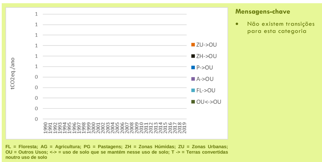
Figura 51: Emissões / Sequestro da Categoria 4F Outros Usos: por subcategoria
