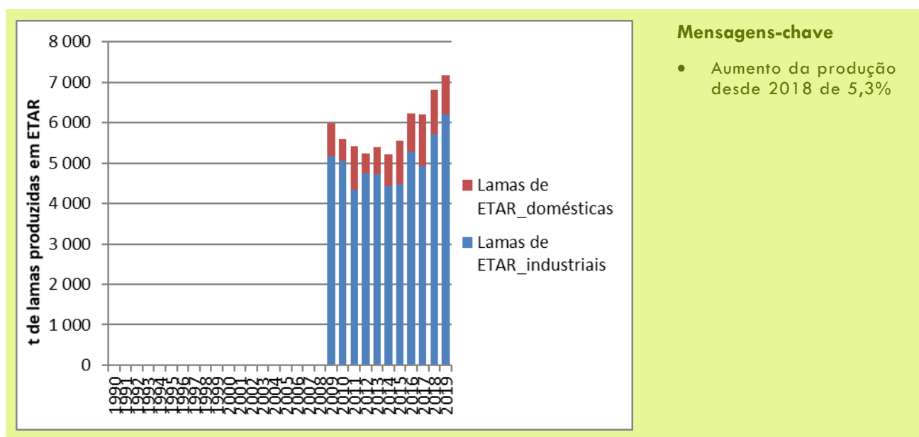
Figura 68: Produção de Lamas de ETAR
