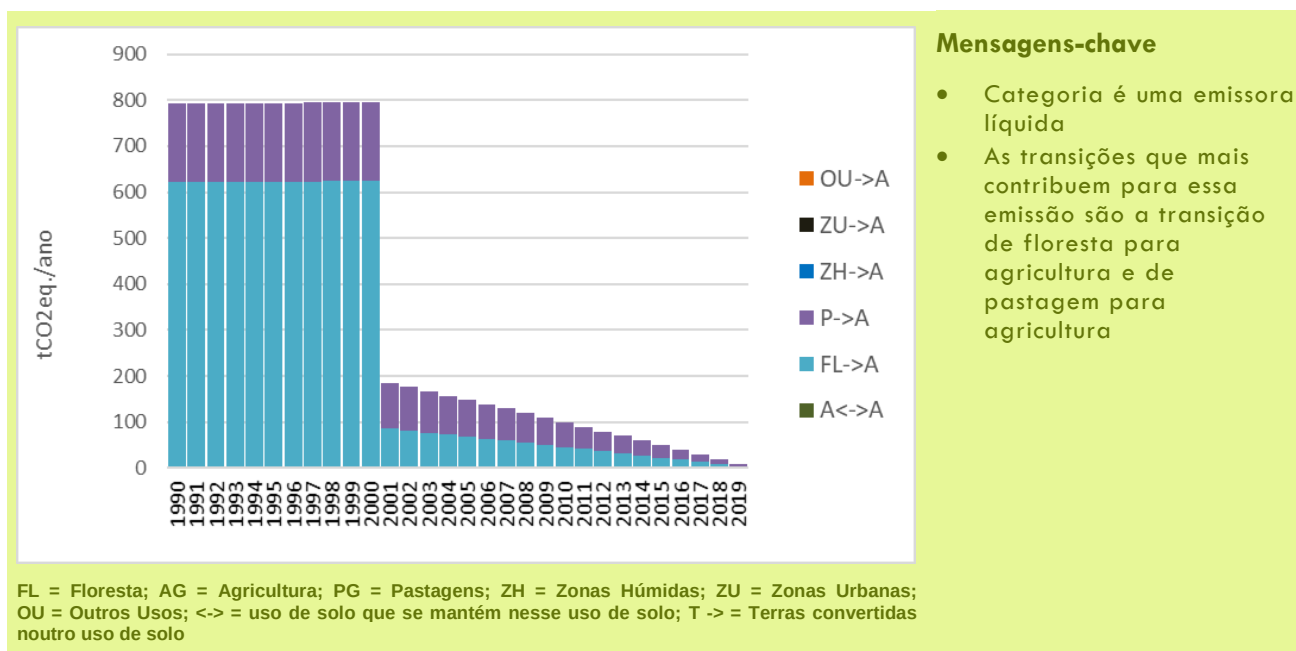
Figura 44: Emissões / Sequestro da Categoria 4B Agricultura: por subcategoria
