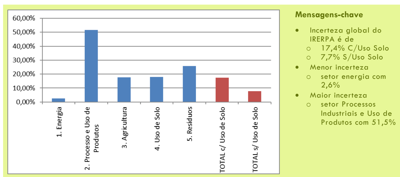
Figura 70: Distribuição da Incerteza do IRERPA por Setor em 2019
