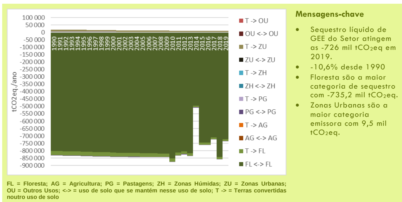
Figura 38: Evolução das Emissões do Setor Uso de Solo, Alterações de Uso do Solo e Florestas
