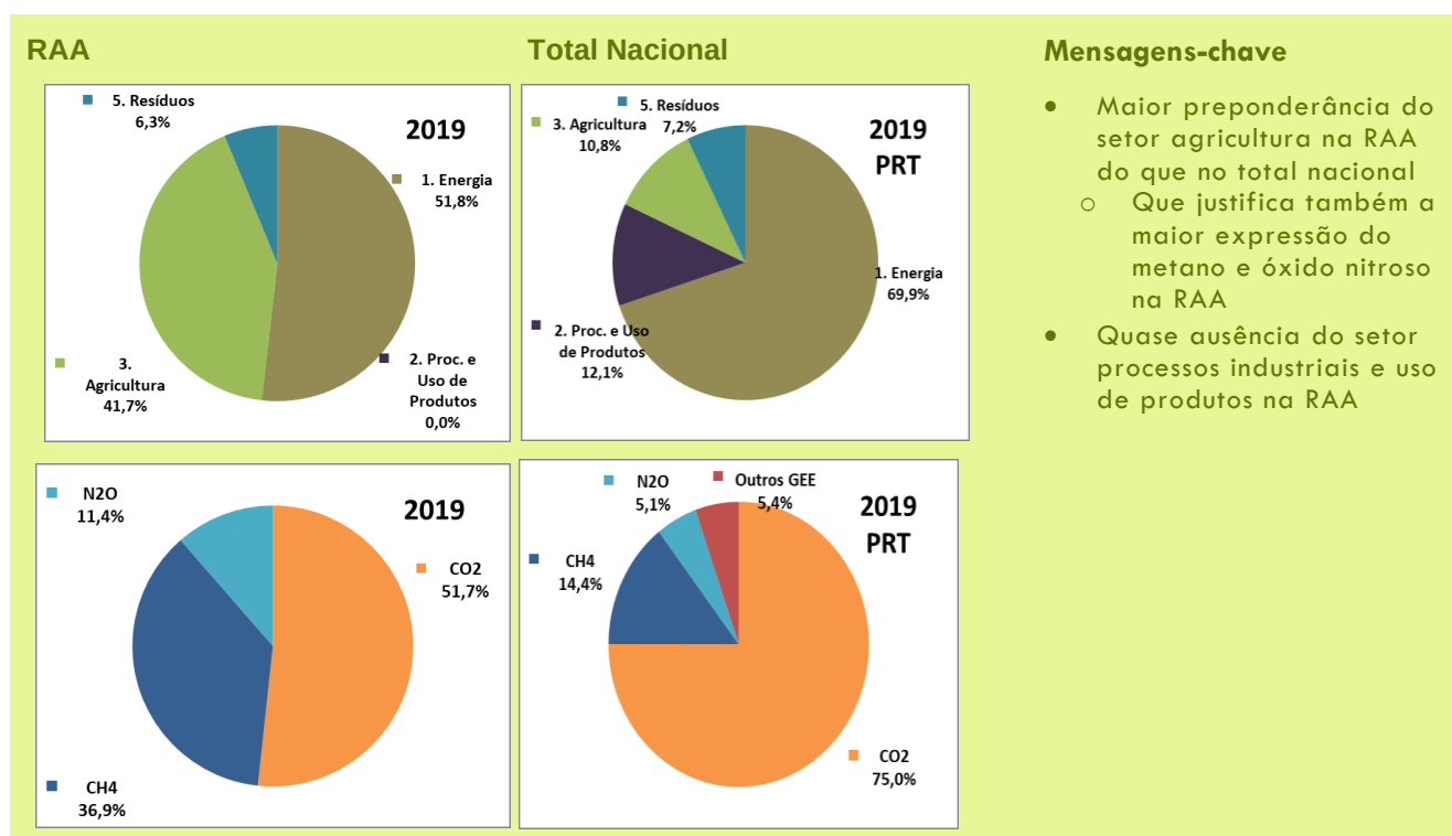
Figura 5: Comparação entre o Perfil de Emissões na RAA e Total Nacional em 2019
