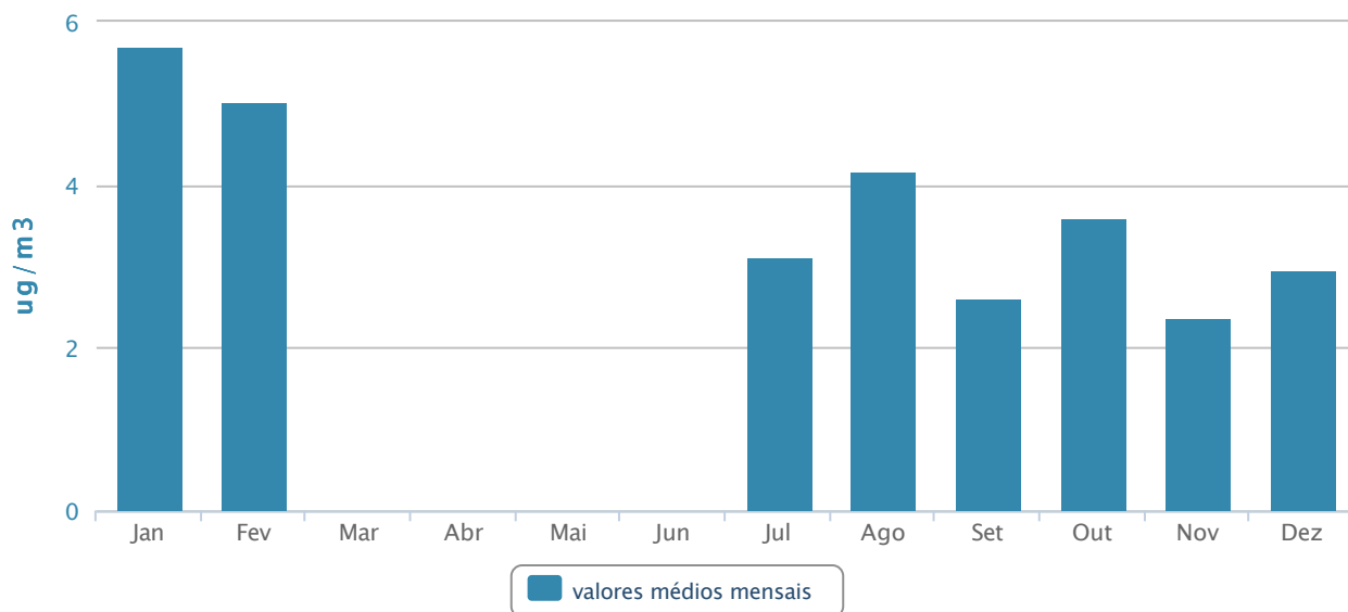
Registos de monitorização de qualidade do ar da Ribeira Grande para o poluente NOx em 2014
