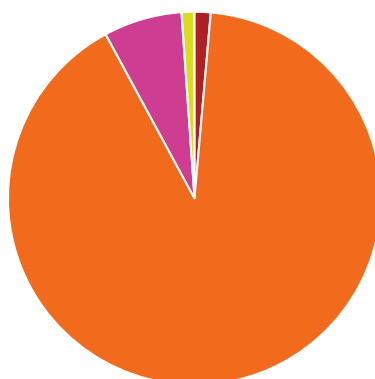
Índice global de qualidade do ar da Região em 2013
