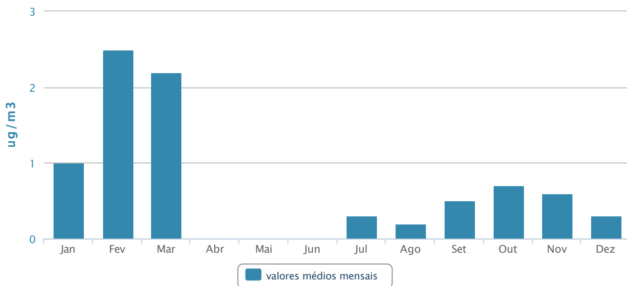
Registos de monitorização de qualidade do ar do Faial para o poluente NO2 em 2014
