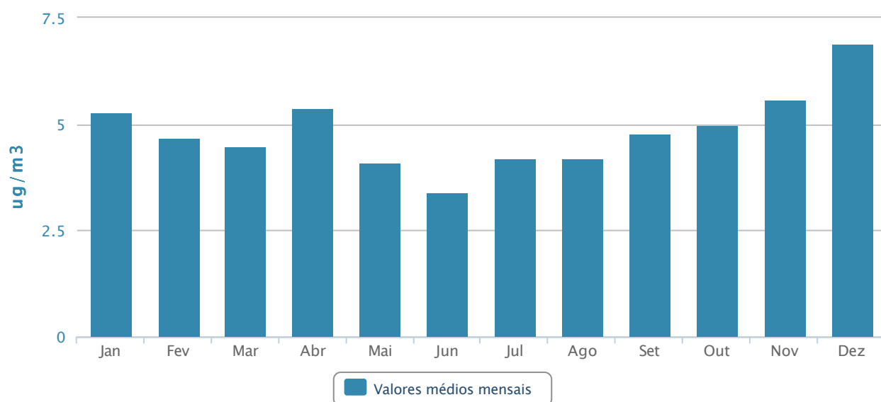
Registos de monitorização de qualidade do ar de Ponta Delgada para o poluente NO2 em 2014
