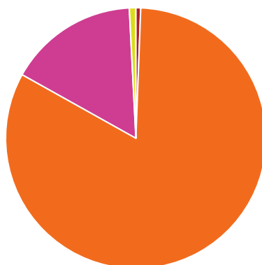
Índice global de qualidade do ar da Região em 2012
