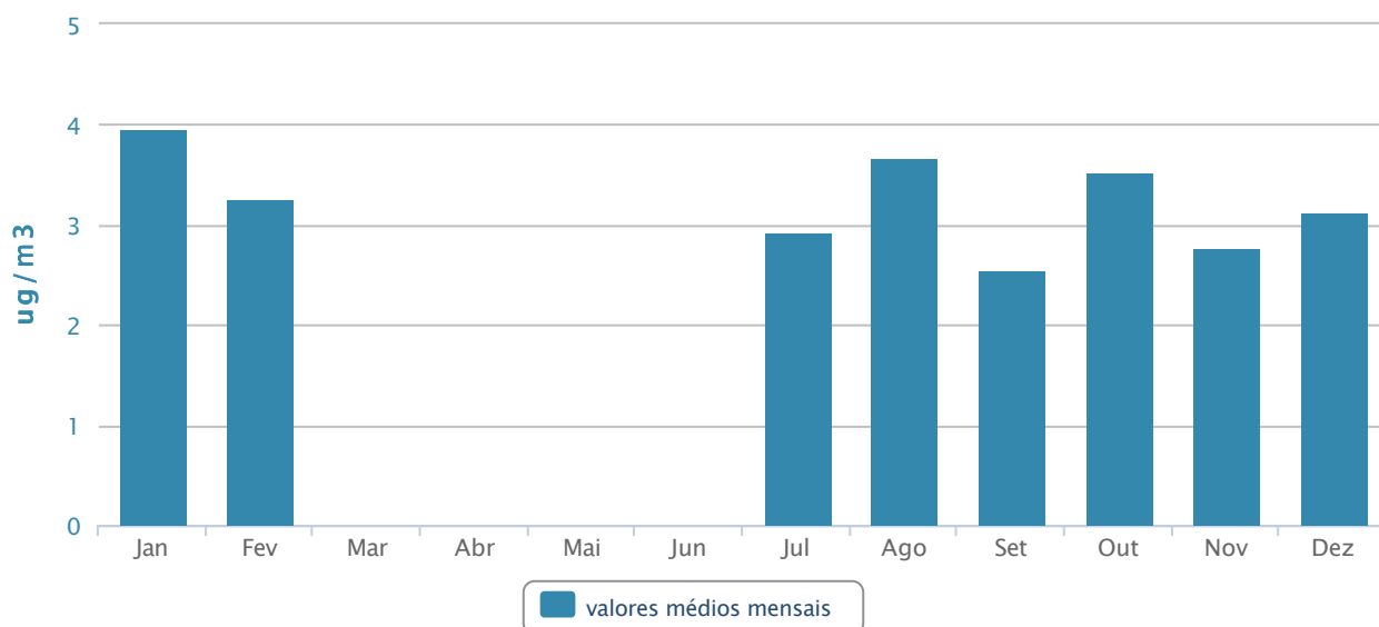
Registos de monitorização de qualidade do ar da Ribeira Grande para o poluente NO 2 em 2014
