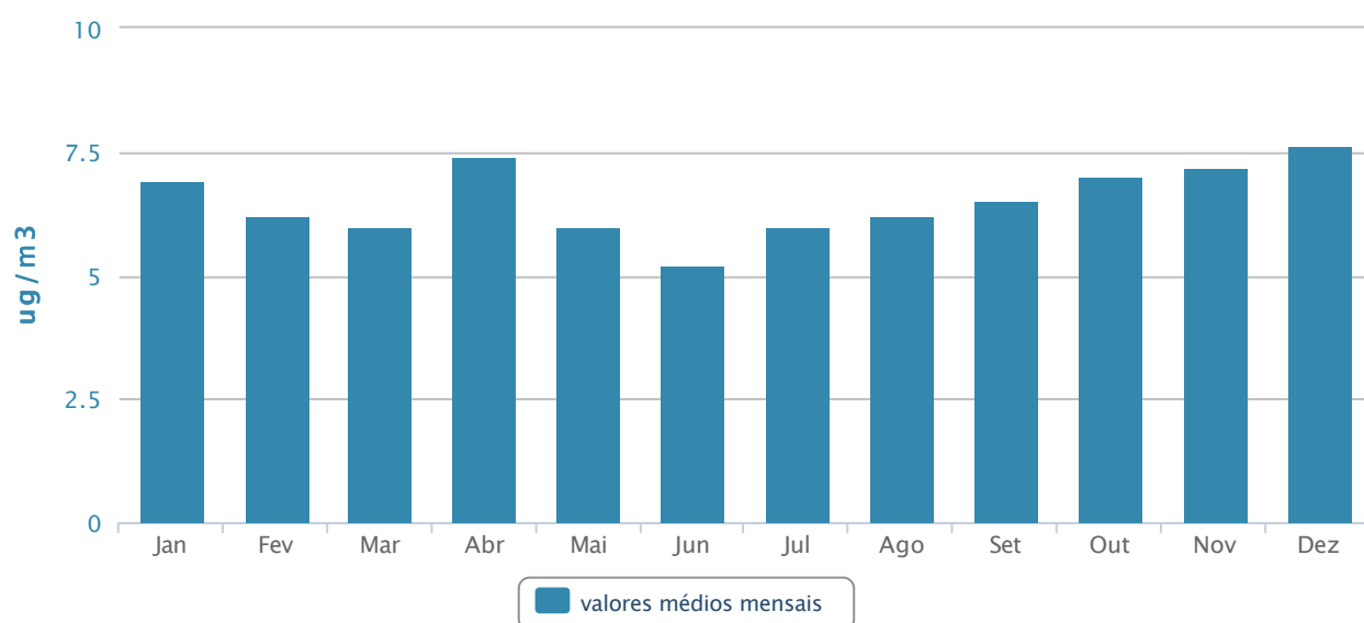
Registos de monitorização de qualidade do ar de Ponta Delgada para o poluente NOx em 2014
